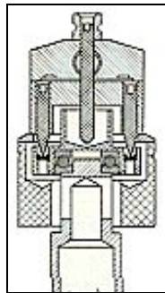
Vue en coupe du DP-6 au niveau du centre des roulements.
